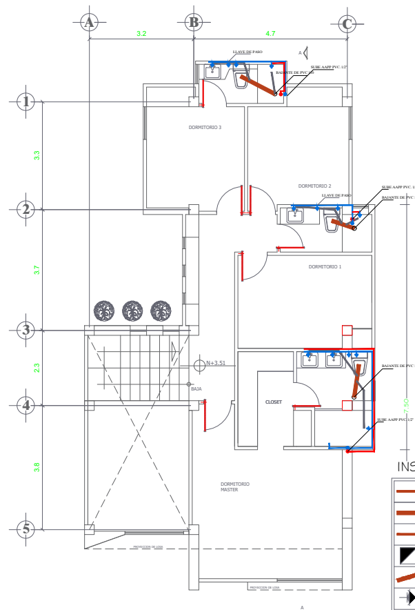
INSTALACIONES SANITARIAS AAPP Y AASS ESCALA: 1:75 PLANTA ALTA
